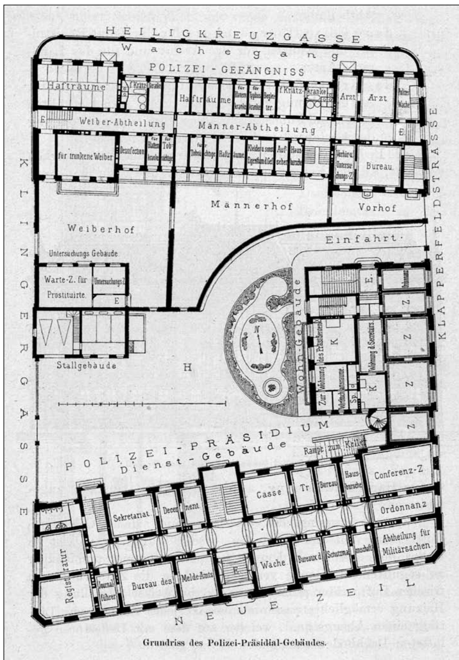
Grundriss des Erdgeschosses des Polizei-Präsidial-Gebäudes, des Dienstwohngebäudes und des Polizeigefängnisses, 1886
